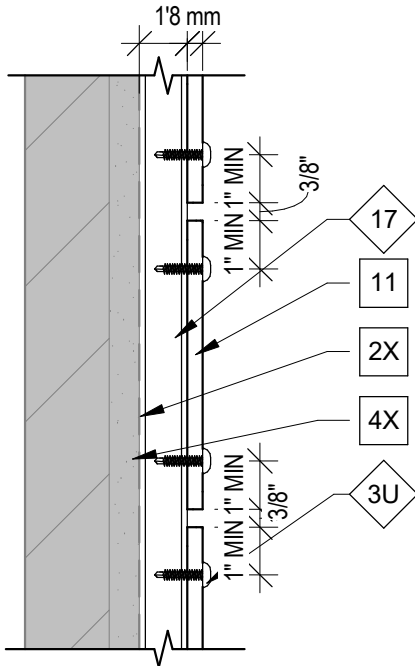
1 INOVEZE E-PLANK HORIZ. JOINT DETAIL O408 SCALE: 3" = 1'-0"
